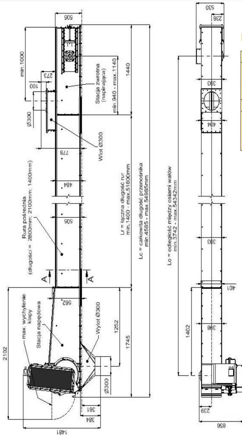
Rys. 2 Przenośnik zabierakowy (redler) Typ PZ150
